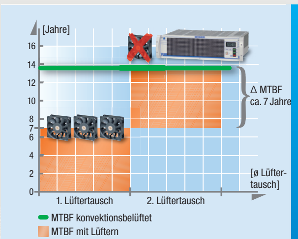
Abb. 3: Die Vorteile der Konvektionsbelüftung des TEBECHOP 4000
