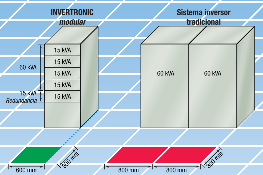
Fig. 6: Comparación de sistemas inversores redundantes n+1
