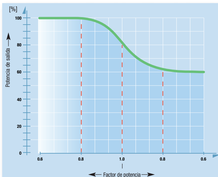
Fig. 8: Potencia aparente del inversor disponible en función del factor de potencia.
