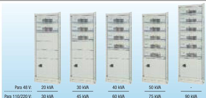
Fig. 9 Regulación del sistema inversor INVERTRONIC modular
